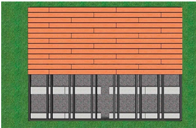
Unterbau, UK und Deck bei 1/3 Längsversatz. Achismaße: 500-117-500-117-500 mm
